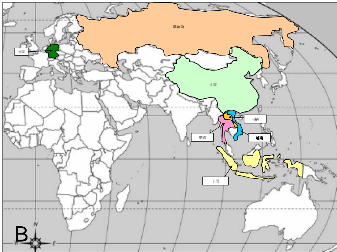
A) 自 2004 年 1 月起於亞洲地區人類感染 H5N1 禽流感的情況(截至 2006 年 9 月 2 日) 及 B) 於 2006 年 8 月 2 日至 2006 年 9 月 2 日期間動物間爆發禽流感的情況。
