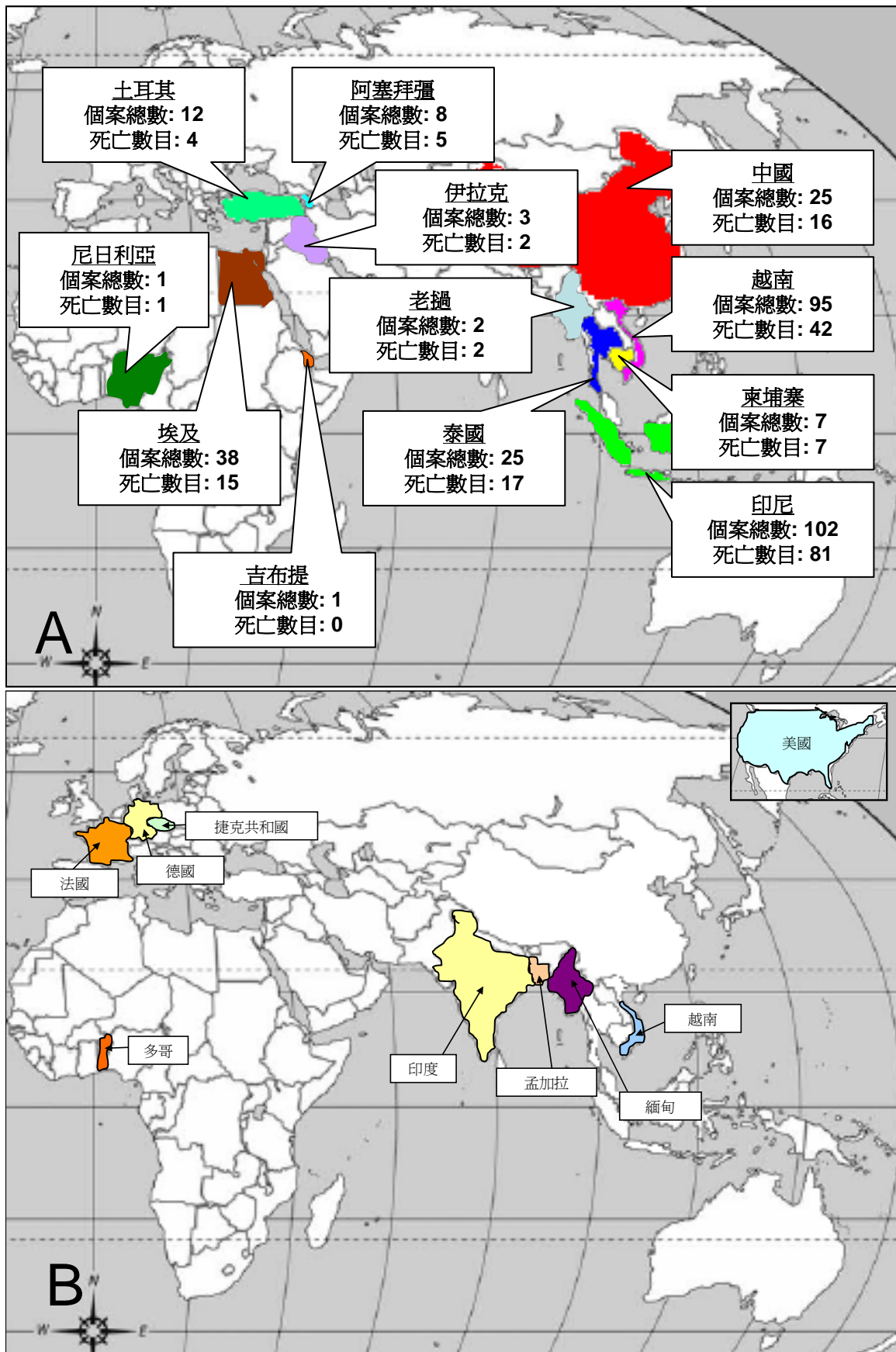
(A) 自 2004 年 1 月起人類感染 H5N1 禽流感的情況(截至 2007 年 7 月 28 日) 及 (B) 於 2007 年 6 月 28 日至 2007 年 7 月 28 日期間鳥類間爆發禽流感的情況。
